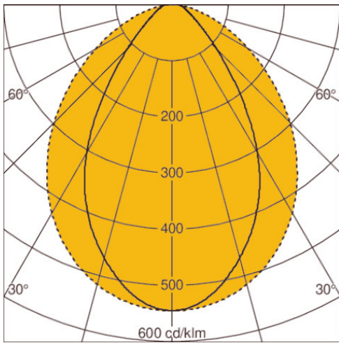
kapea valonjako
