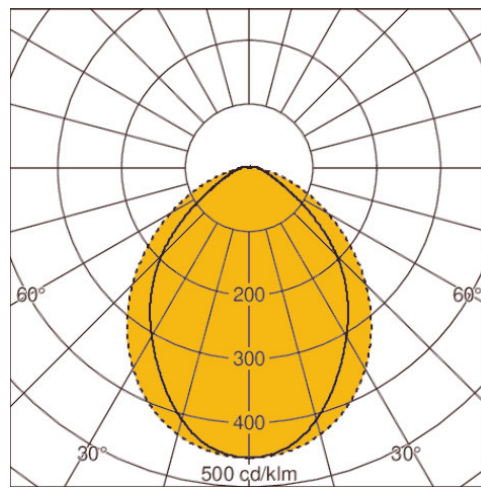
keskileveä valonjako
