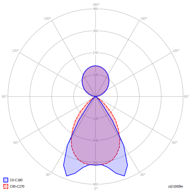
Suora/epäsuora valonjako - lamellitilä/opaali
