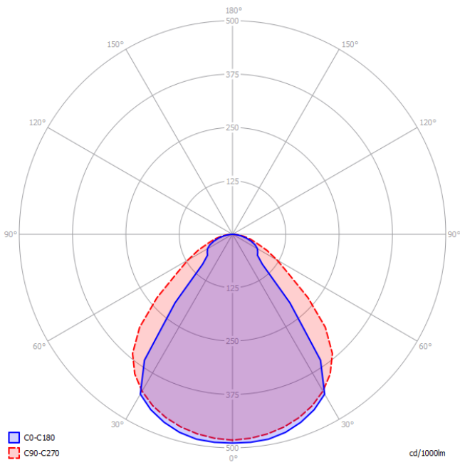
Suora valonjako - mikroprisma
