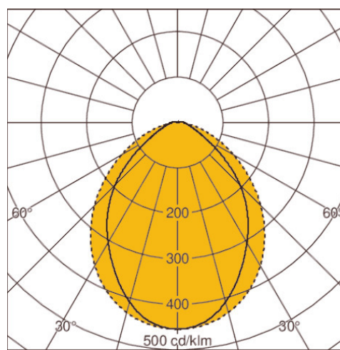
keskileveä valonjako
